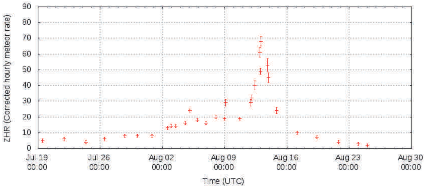
FIGURA 3. Perfil de actividad de las Perseidas del pasado 2014 con todas las observaciones remitidas a la International Meteor Organization. La actividad máxima alcanzada fue de unos 65 meteoros (en Tasa Horaria Zenital) Nótese que ese año hubo Luna Llena, de modo que muchos meteoros débiles no se observaron.
