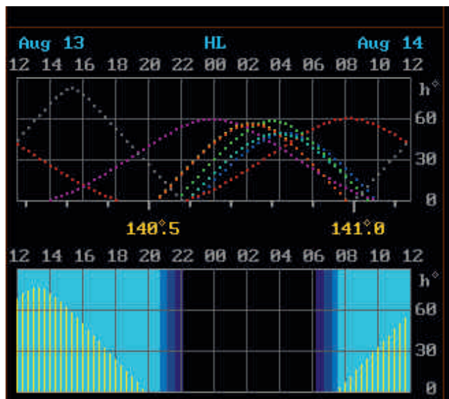
CONDICIONES DE VISIBILIDAD DESDE CANARIAS.
