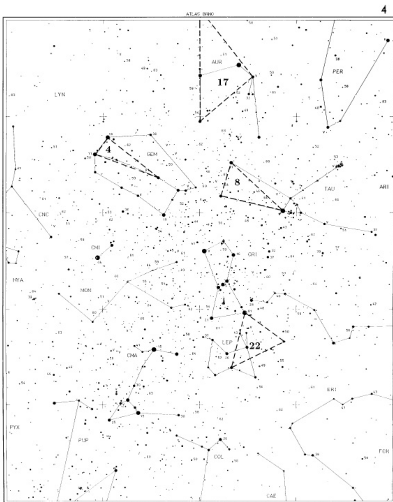
FIGURA 5. Carta 4 del atlas BRNO ( http://www.imo.net/docs/images/4a-260.png ) donde se muestran las áreas de MALE adecuadas en la observación de meteoros.
