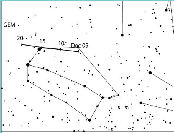
FIGURA 1. Desplazamiento aparente del radiante de las Gemínidas. La observación visual hay que hacerla a unos 30 grados de esa posición.
